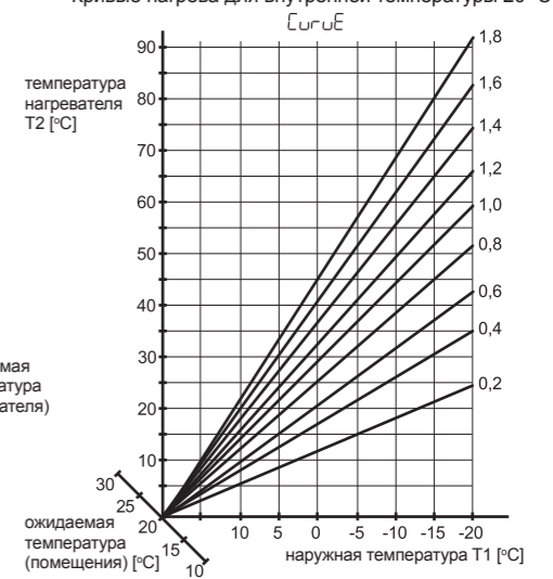
Кривые нагрева для внутренней температуры 20 °C
